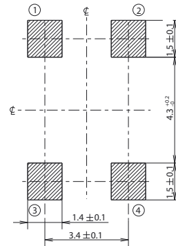
P.C.B. LAYOUT
